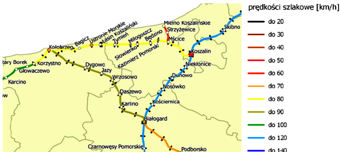
Rycina 42. Prędkości szlakowe dla składów wagonowych (stan na 12.2013 r.)
